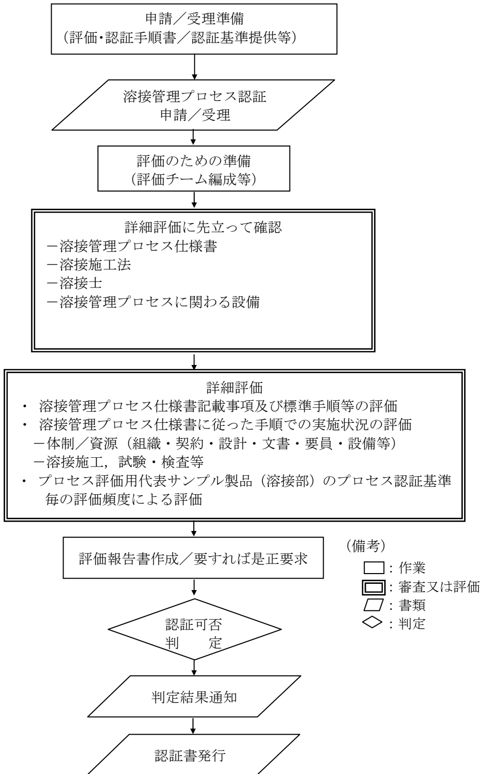
付表 1 溶接管理プロセス評価・認証の概略フロー
