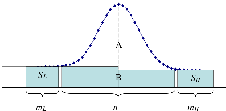
15 図3 段差のベースラインを仮定したピーク面積の求め方
