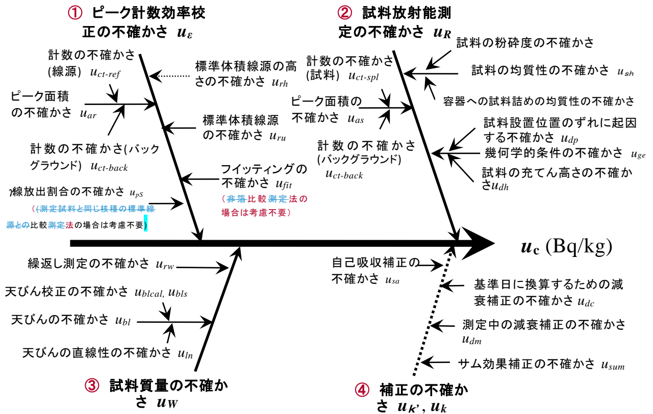
図2 ガンマ線スペクトロメトリーによる放射能濃度測定の不確かさの特性要因図(例)
