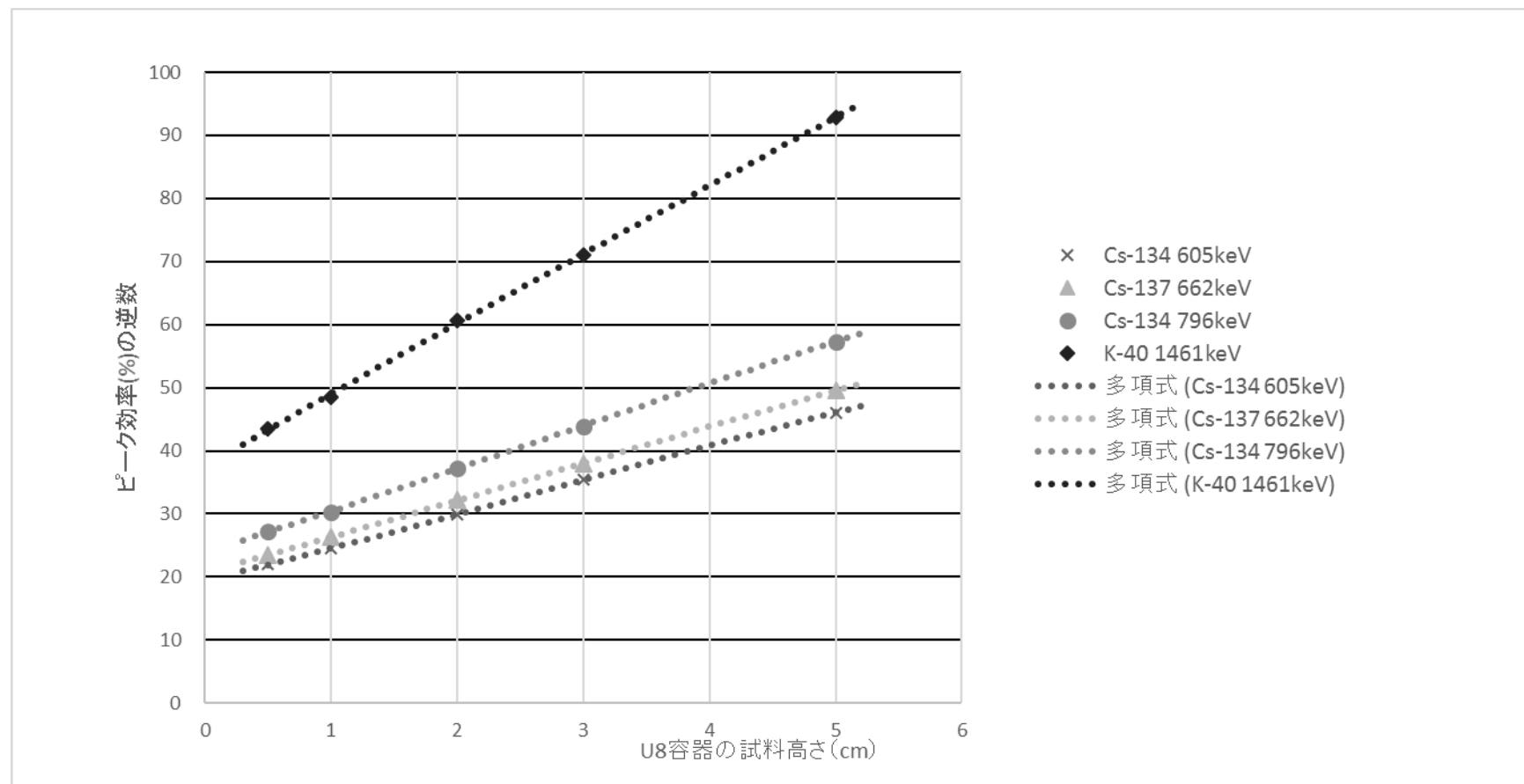
図5 U8 容器の試料高さ とピーク効率の関係
