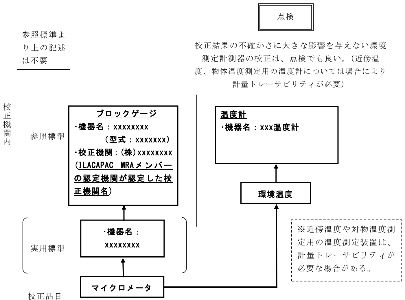
計量トレーサビリティ体系図 例 1. 国家標準がある場合の校正機関
